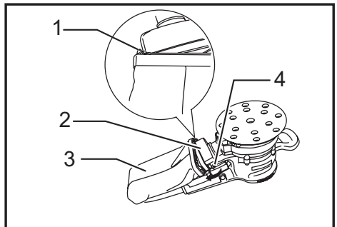
► 1. Hook 2. Dust nozzle 3. Dust bag 4. Push button
