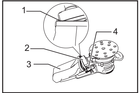
► 1. Gancho 2. Boquilla para polvo 3. Bolsa para polvo 4. Botón pulsador
